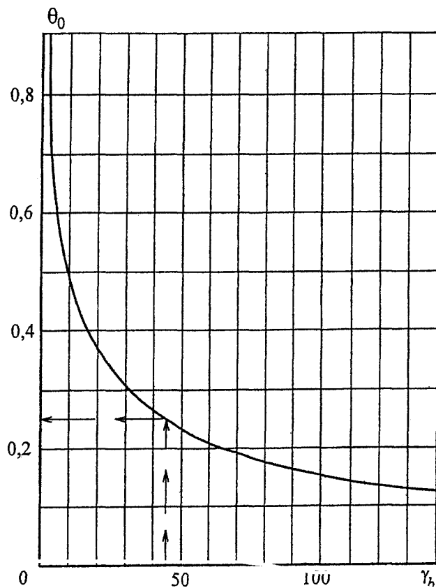
Рисунок М.1. График для определения \theta_0
