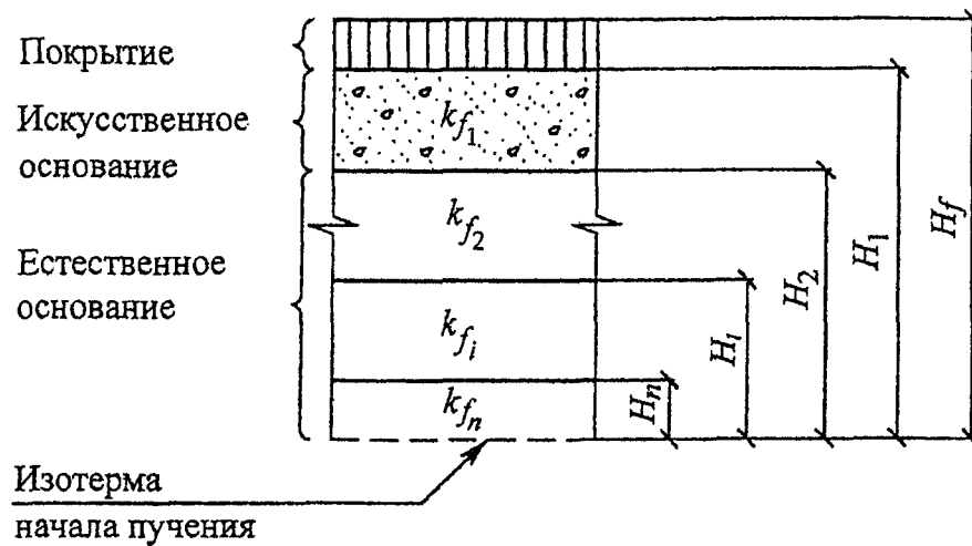
Рисунок Е.1. Расчетная схема слоистого основания
