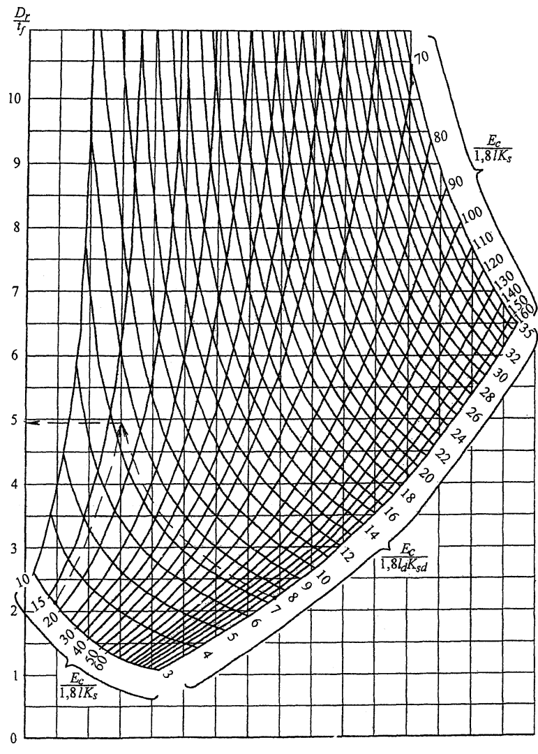
Рисунок М.2. Номограмма для определения соотношения \frac{D_r}{t_f}
