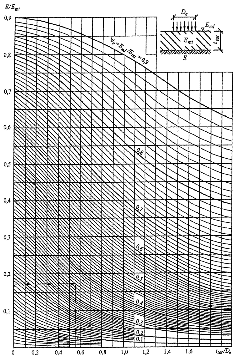
Рисунок К.4. Номограмма для определения коэффициента \psi_k
